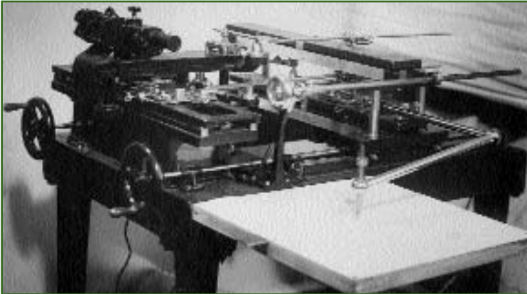
Рис. 4 Стереоавтограф
